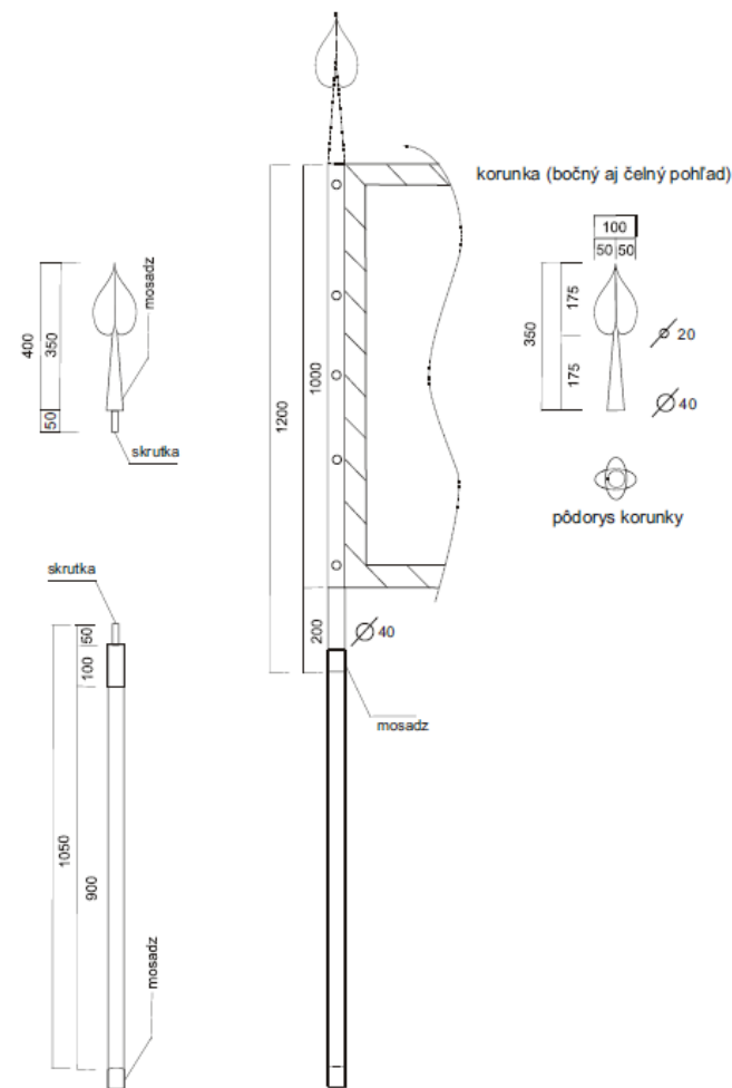
konštrukcia žrde
