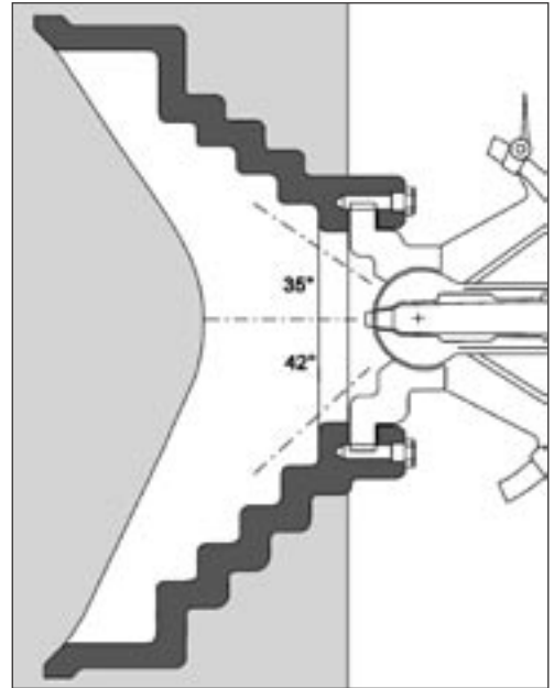
Půdorys širší střelny pro lafetu DZ 10. (výkres Martin Dubánek)
