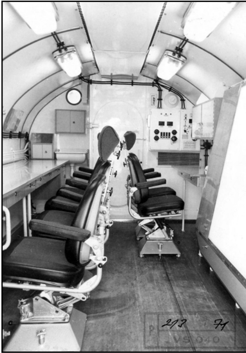
8) Interiér funkčného vzorku VESTA C v roce 1971. (foto VHA)
