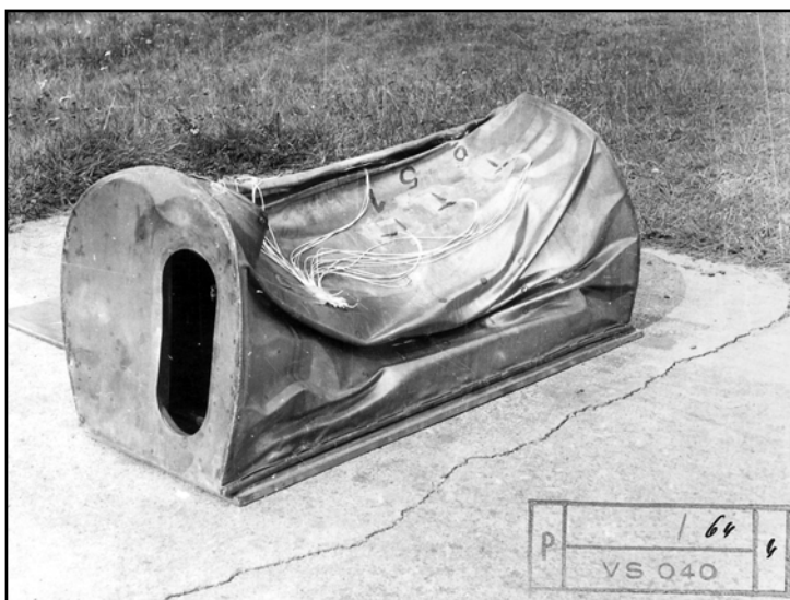
3b) Deformační zkoušky modelů úkrytu VESTA-B v Borečku u Mimoně v roce 1964. (foto VHA)
