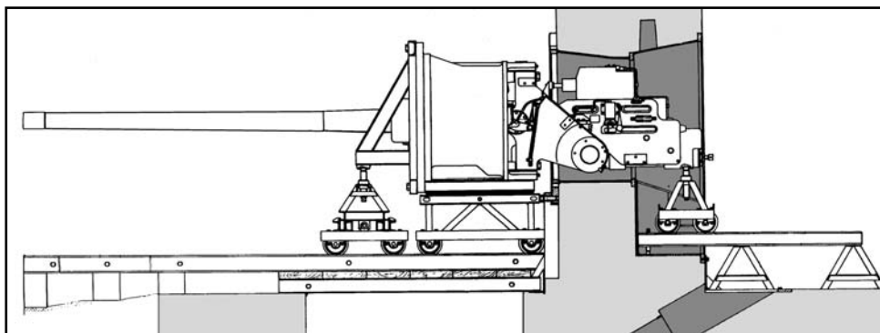
5) Schéma instalace 85mm kanónu vz. 44/59 do střelny pomocí tzv. přetahovacího zařízení. (podle Dě1-21-11 upravil autor)
