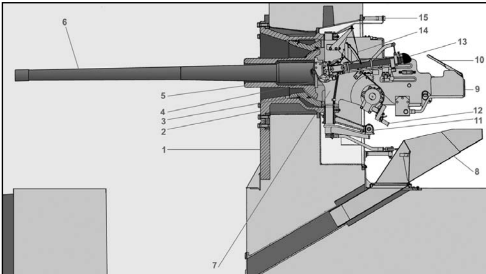
3) 85mm pevnostní kanón vz. 44/59:1 rám střelny, 2 rám (lafety), 3 clona, 4 kolébka, 5 pancíř kanónu, 6 hlaveň, 7 nosič kolébky, 8 odvod nábojnic, 9 lapač nábojnic, 10 nabíjecí žlab, 11odměrové řídicí, 12 náměrové řídicí, 13 záměrný dalekohled, 14 pomocný zaměřovač, 15 ukazatel odměru. (podle Dě1-21-11 upravil autor)
